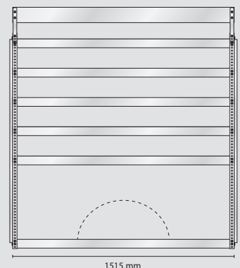
S118 Gewicht 36,8 kg
