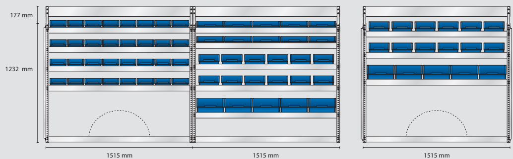
S91 poids 42,9 kg
